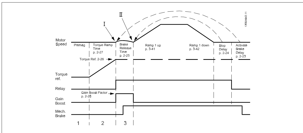
Рисунок 2.4: Последовательность отпущания тормоза при управлении механическим тормозом подъемного механизма
